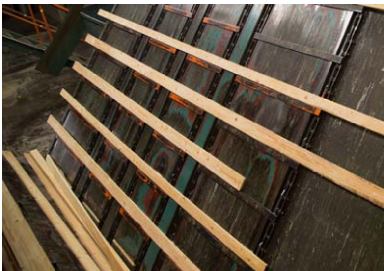
Enstycksmatning av brädor mellan kantning och paketläggning.
